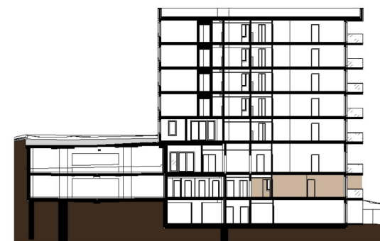
ŘEZ OBJEKTEM
