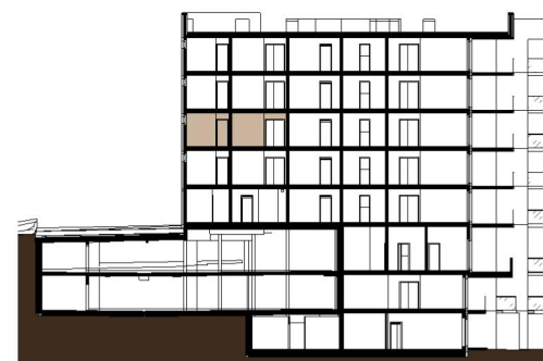
ŘEZ OBJEKTEM
