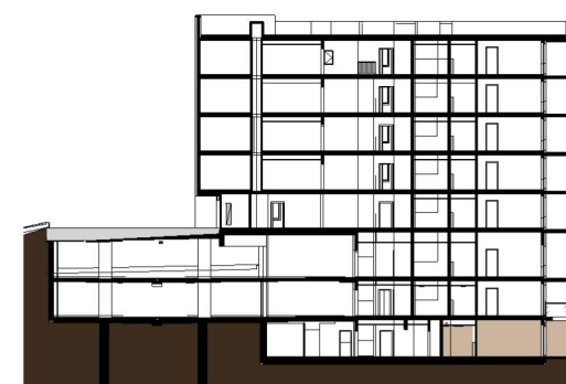
ŘEZ OBJEKTEM
