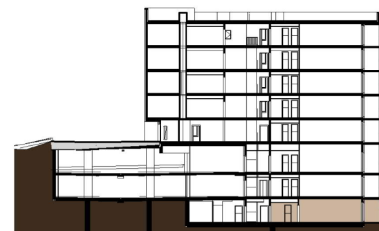
ŘEZ OBJEKTEM
