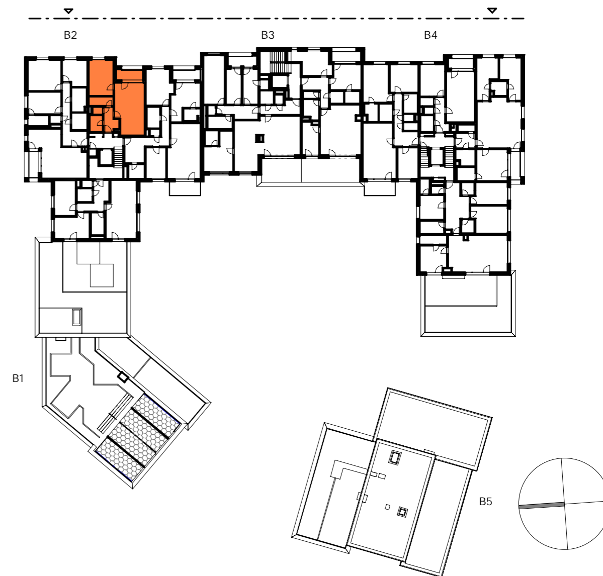
PŮDORYS 5.NP
