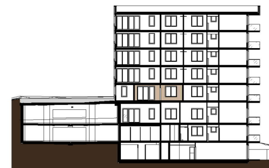
ŘEZ OBJEKTEM
