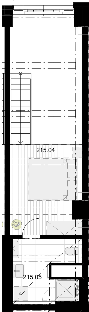
PŮDORYS 2.NP LOFT horní podlaží
