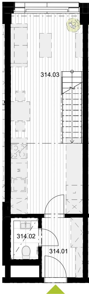
PŮDORYS 3.NP spodní podlaží
