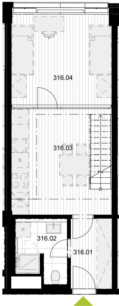
PŮDORYS 3.NP spodní podlaží
