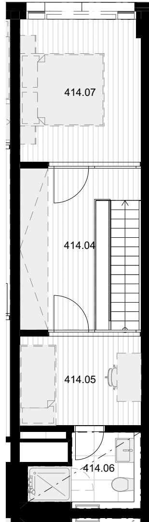
PŮDORYS 4.NP LOFT horní podlaží
