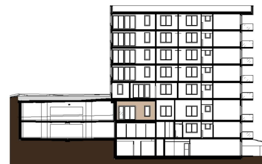
ŘEZ OBJEKTEM
