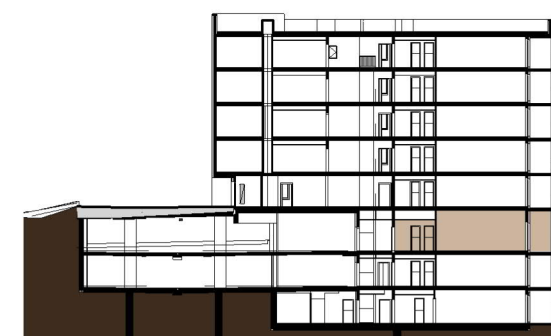
ŘEZ OBJEKTEM
