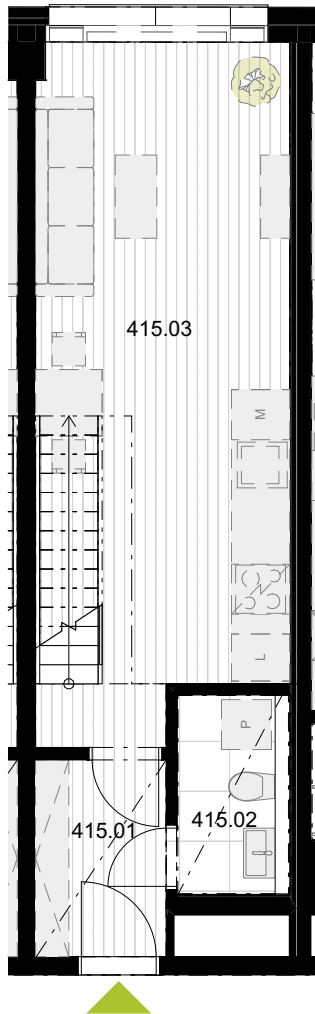
PŮDORYS 4.NP spodní podlaží
