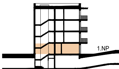
ŘEZ
