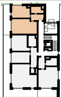
PŮDORYS PATRA
