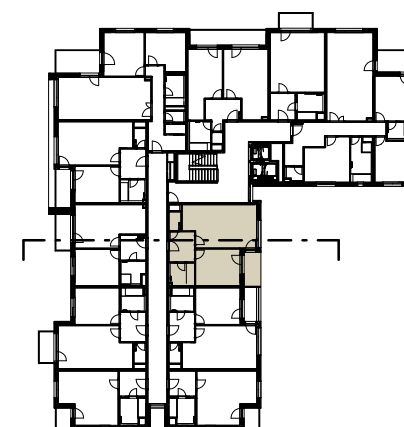
PŮDORYS PODLAŽÍ
