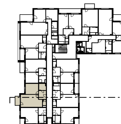
PŮDORYS PODLAŽÍ
