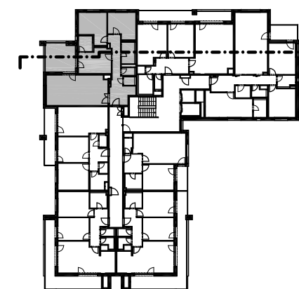
PŮDORYS PODLAŽÍ
