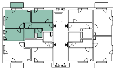
Schéma podlaží
